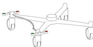
Roues Ø125 à freinage centralisé, sur les côtés (gauche, droite ou les deux)
